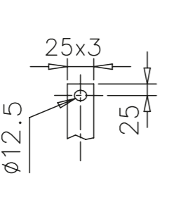
HV Terminal
